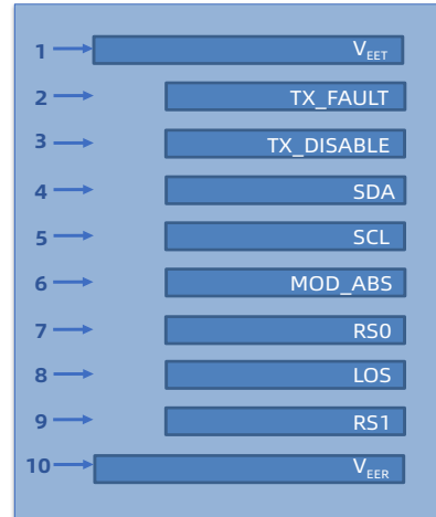
底部直视图
