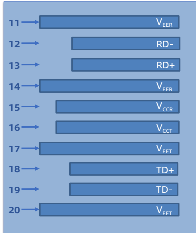
顶部直视图
