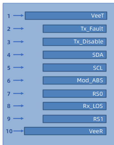
底部视图
