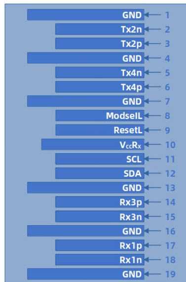
底部视图
