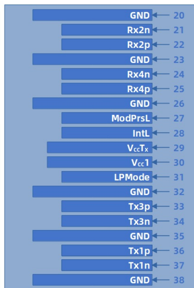
顶部视图
