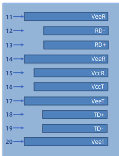
顶部视图
