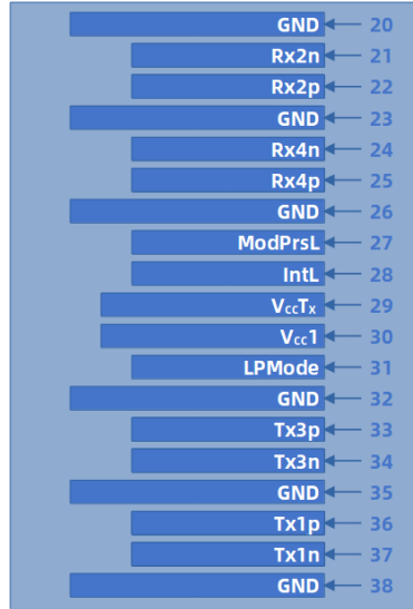
顶部直视图
