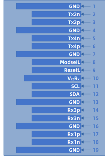
底部直视图
