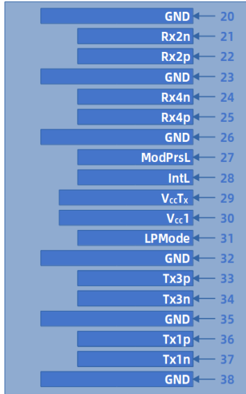
顶部视图
