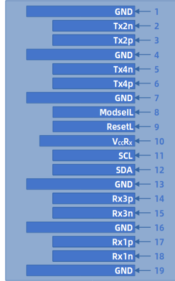
底部视图
